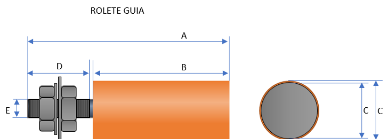
Figura 3 - Rolos Guia
