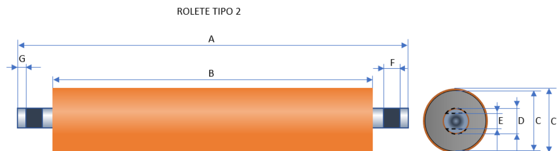
Figura 2 - Rolos de Roletes do tipo 2
