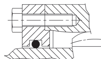
Detalhe "X": Construção de tampas para tamanhos LFG – 111 e maiores.
