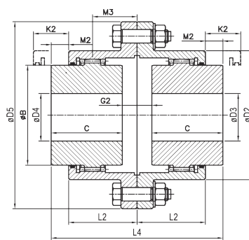
Acoplamento AGD com dois Cubos Reversos
