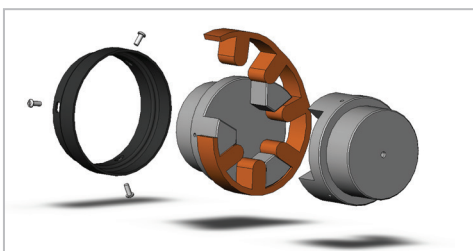
SW95 ao SW225 PU
