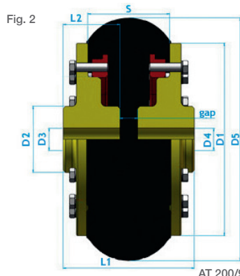
CUBOS CE II
