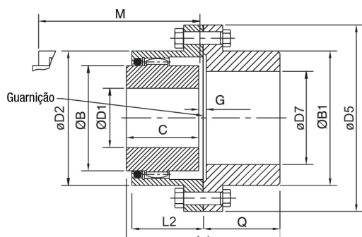
TIPO LHG (simples engrenamento)
