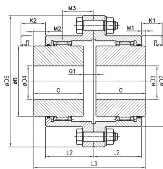
Acoplamento AGD com um Cubo Reverso
