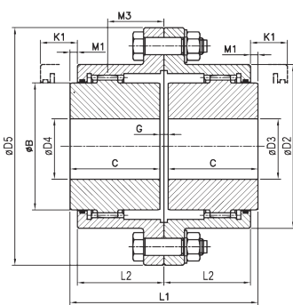
Acoplamento AGD
