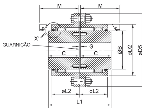
TIPO LFG (duplo engrenamento)
