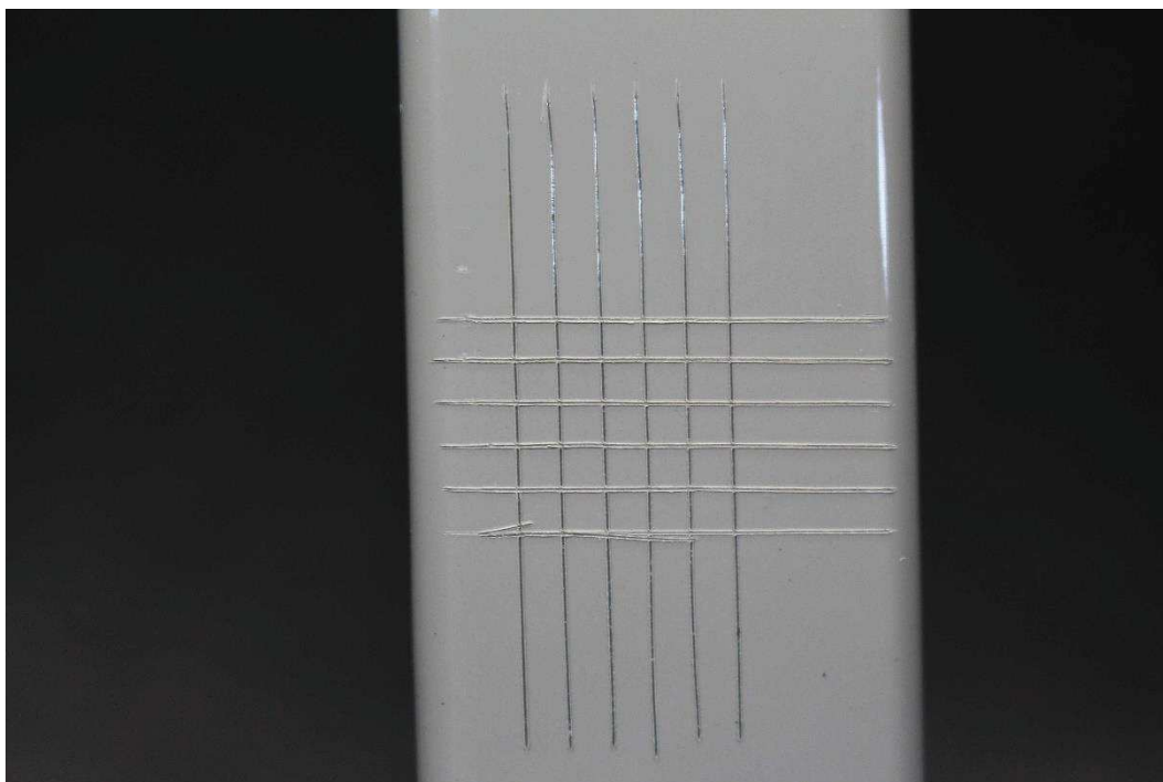
CP 3 após teste de aderência. Detalhe de teste 2.
