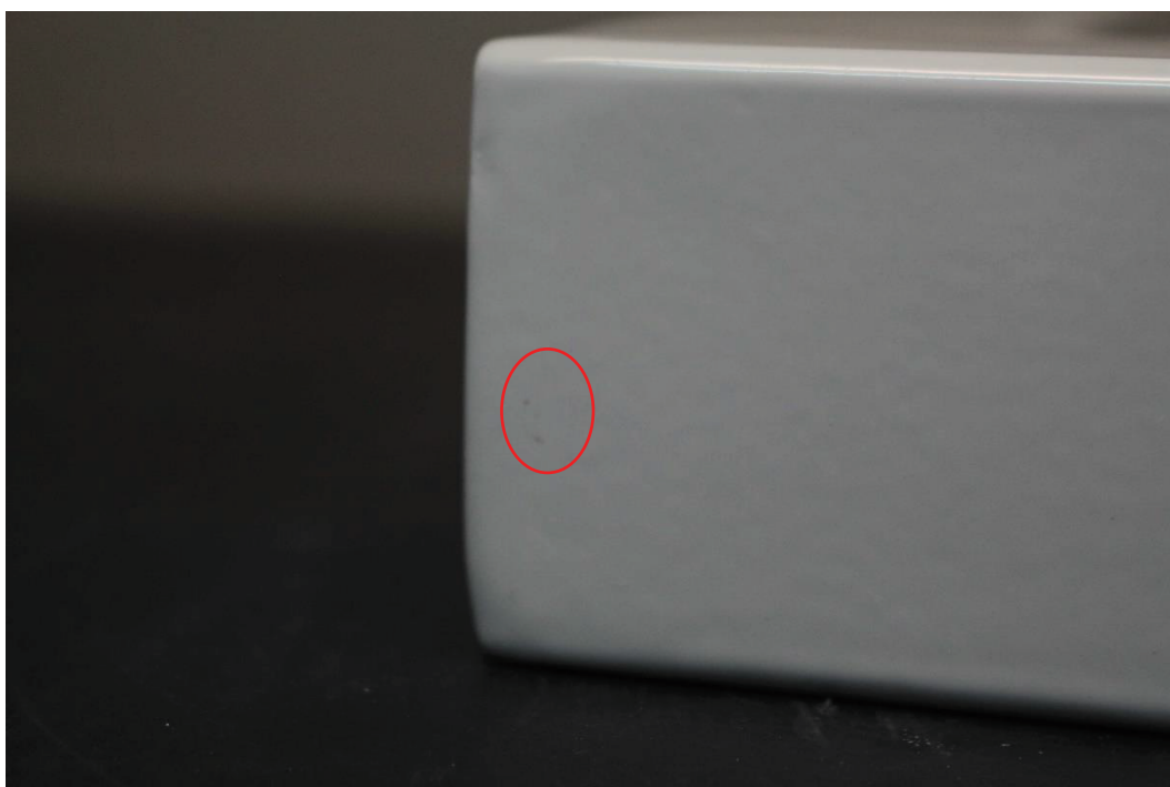
Amostras 2 após 672 horas. Ponto de corrosão vermelha.
