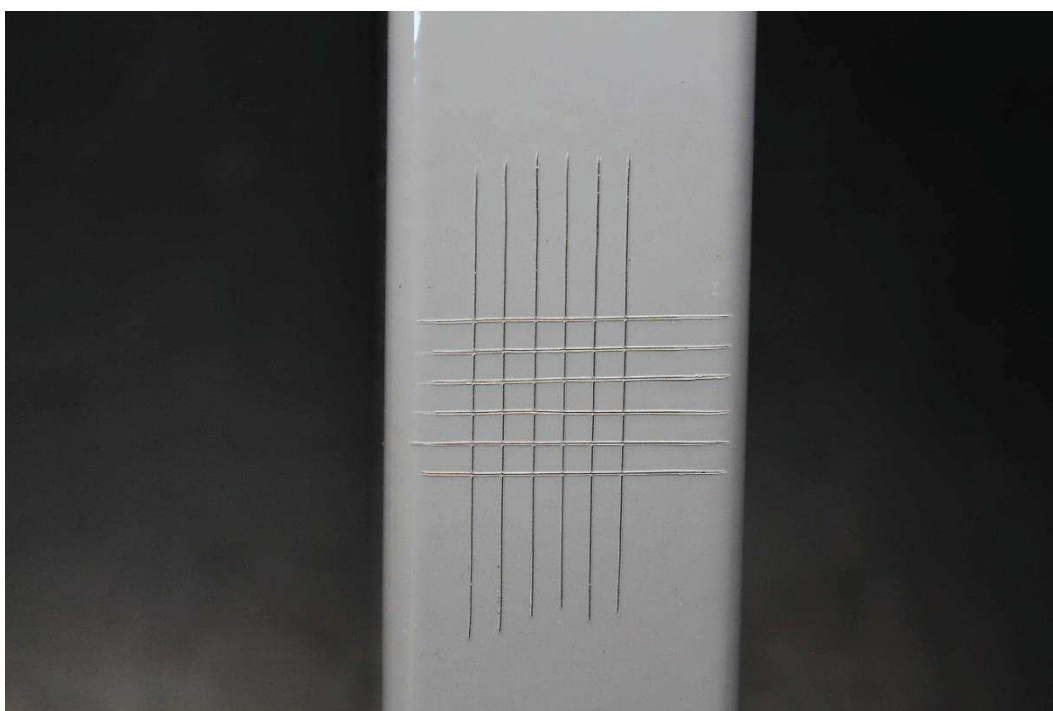
CP 2 após teste de aderência. Detalhe de teste 2.
