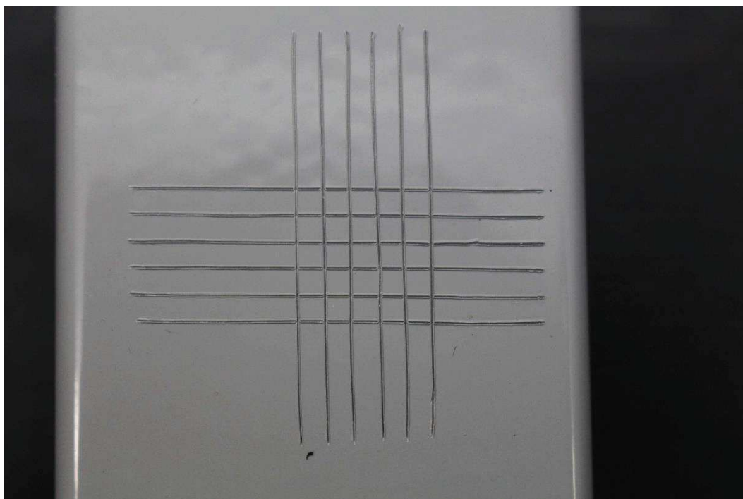
CP 2 após teste de aderência. Detalhe de teste 1.
