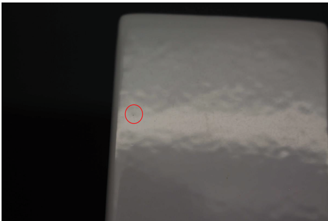
Amostras 1 após 672 horas. Ponto de corrosão vermelha.
