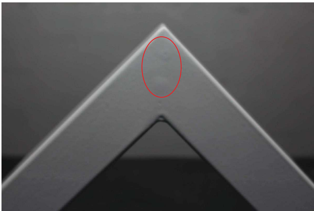
Amostras 1 após 672 horas. Bolhas.
