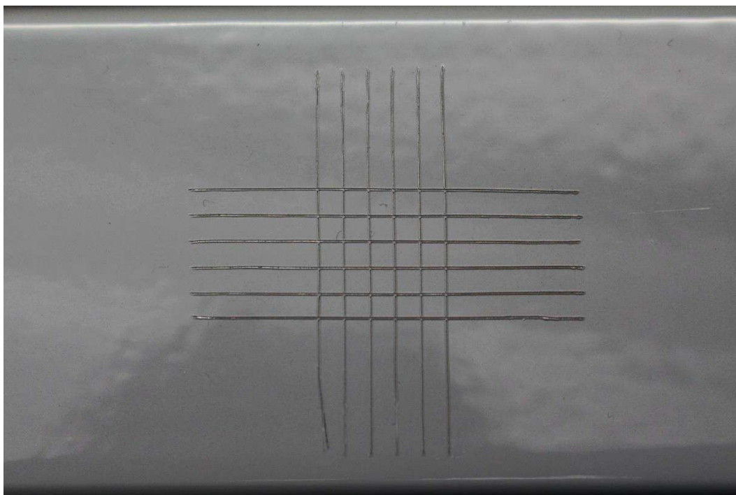
CP 2 após teste de aderência. Detalhe de teste 3.
