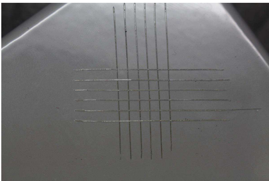
CP 3 após teste de aderência. Detalhe de teste 1.
