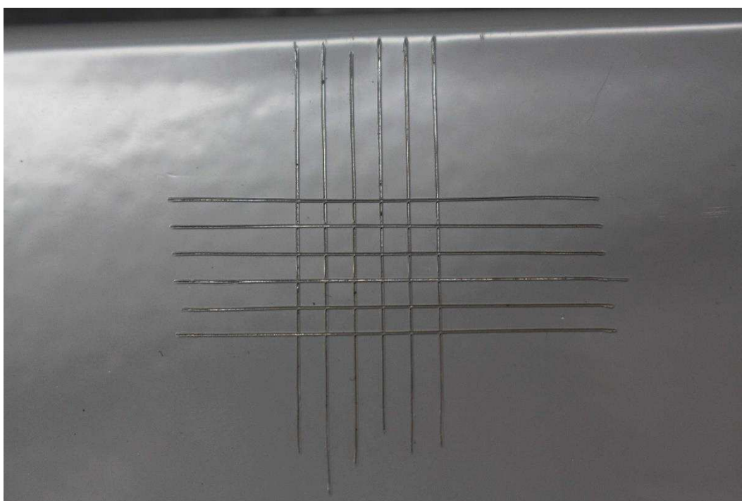
CP 3 após teste de aderência. Detalhe de teste 3.
