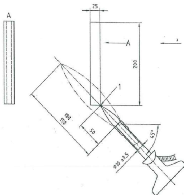
Imagem da configuração do queimador a gás e da peça de teste durante o teste.
