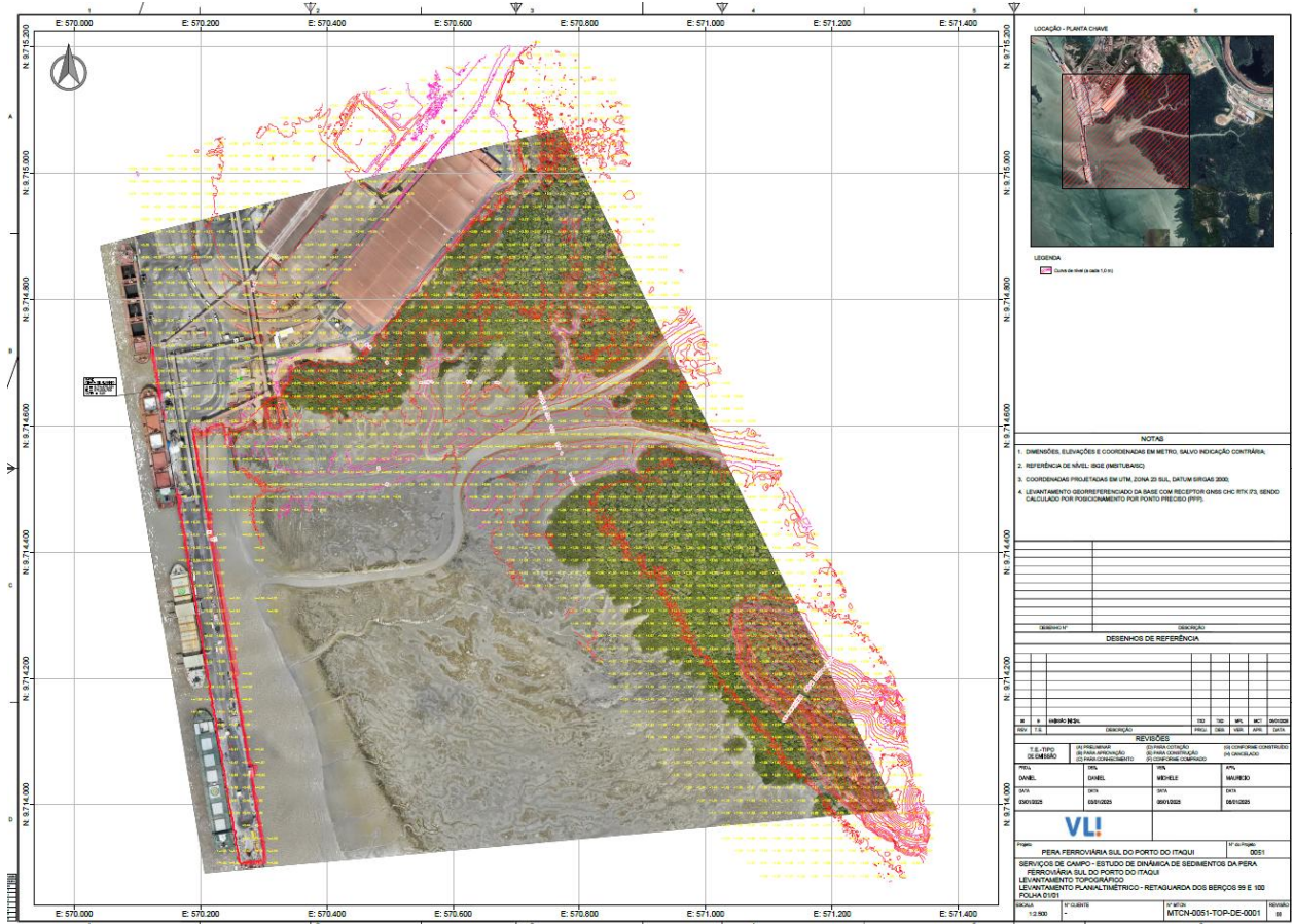
Figura 3 – Planta topográfica.
